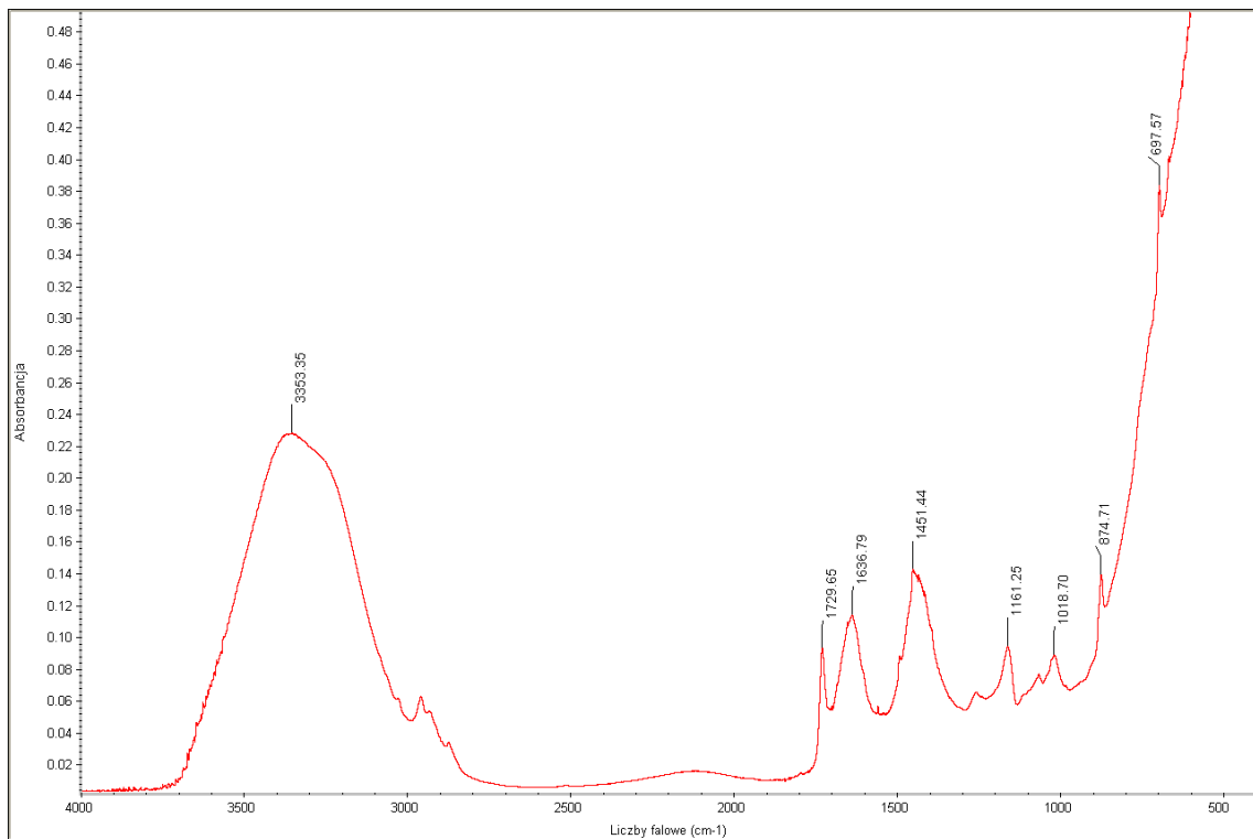
Rysunek Z-2 - Widmo w podczerwieni materiału Akrylit 3000 Siloxan
