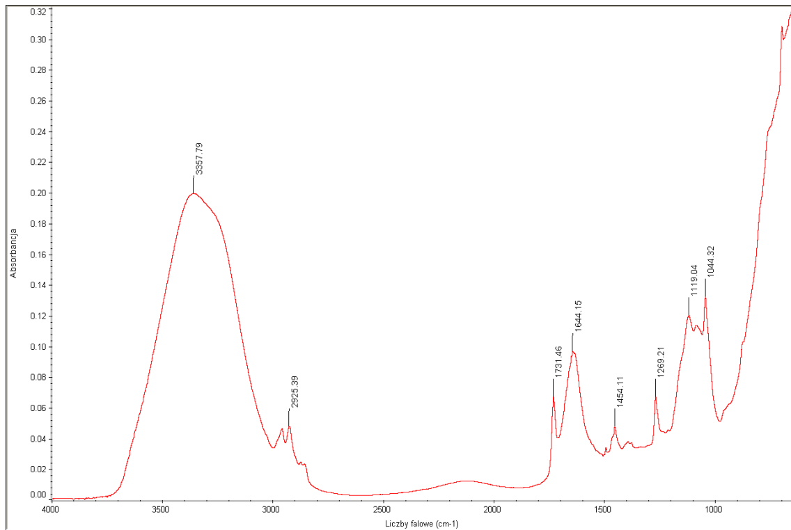
Rysunek Z-1 - Widmo w podczerwieni materiału Bloker
